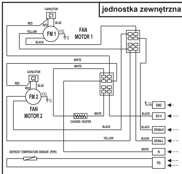
AERO - 15 (DC)
