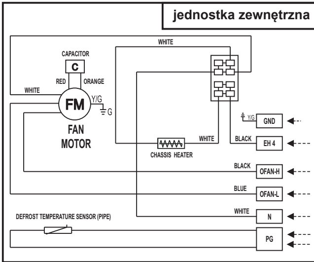
AERO - 7 (DC)
