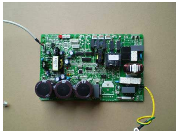
Płyta główna
