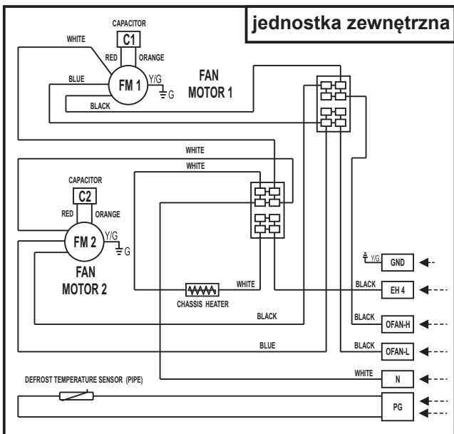
AERO - 12 (DC)
